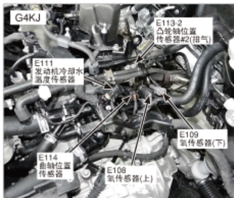
19.发动机后部
