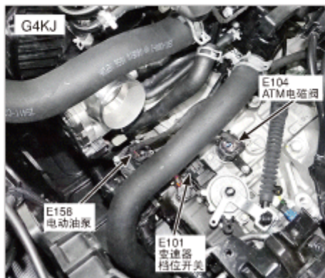
20.变速器顶部
