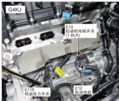
22.发动机左侧
